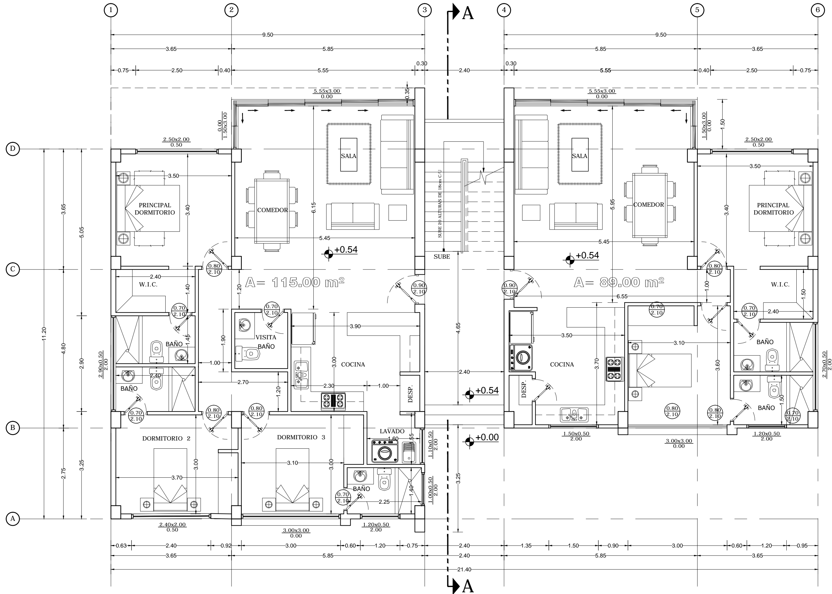
PLANTA BAJA
